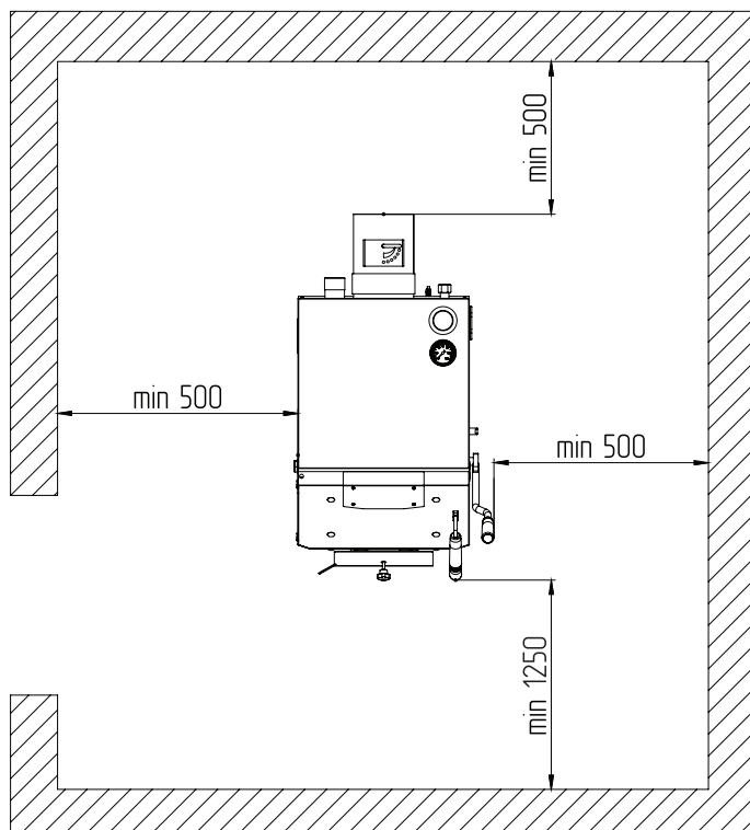
Рис.2 Расположение котла в помещении котельной
